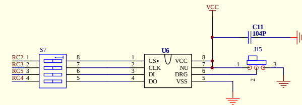
93CX SPI EEPROM
