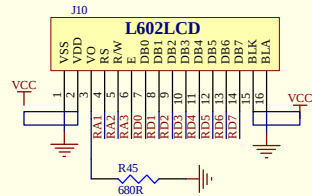
LCD1602
