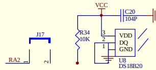
DS18B20
