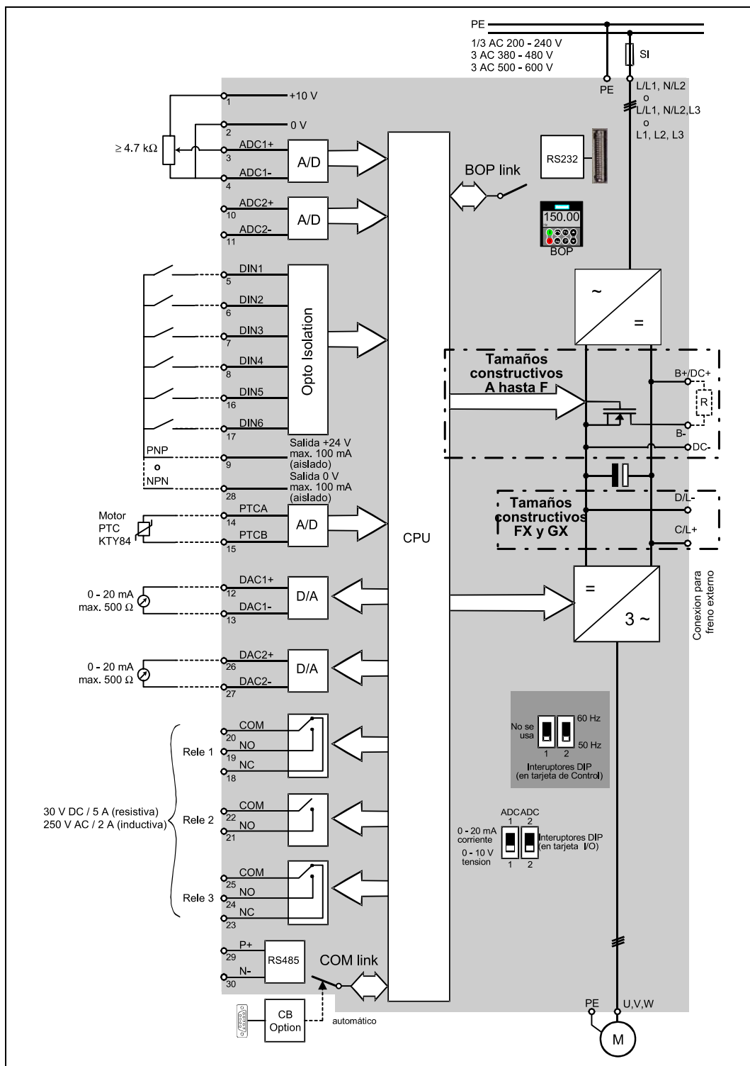
Figura 3-16 Diagrama de bloques MICROMASTER 440
