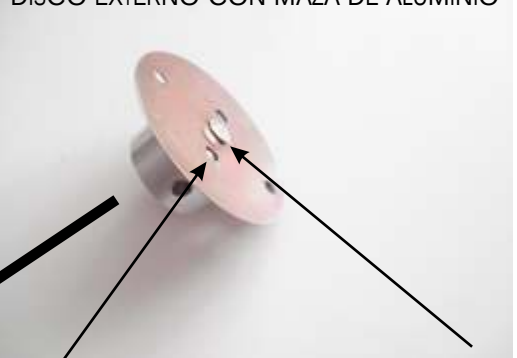
DISCO EXTERNO CON MAZA DE ALUMINIO
